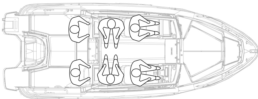
Figur 4.1 Cross 60 Cabin seter for maksimalt seks (6) passasjerer
