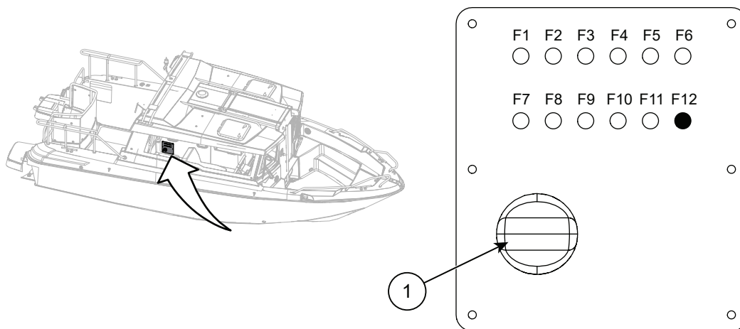
Figur 8.1 Cross 60 Cabin hovedbryter og sikringspanel
