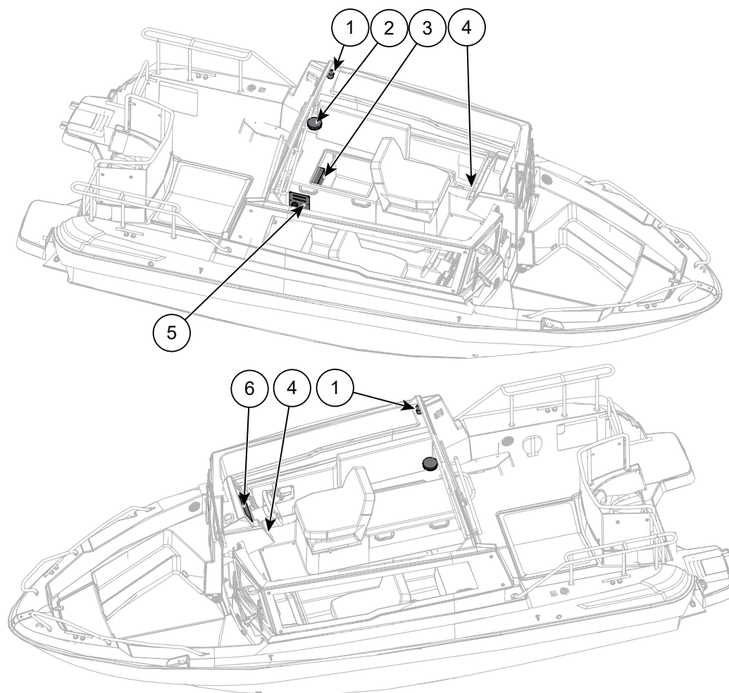
Figur 8.3 Cross 60 Cabin elektrisk utstyr
