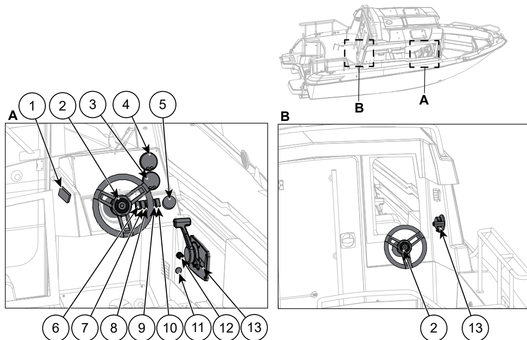
Figur 5.1 Styrestasjonskontroller i kabinen (A) og utvendige styrestasjonskontroller (B) tilgjengelig som ekstrautstyr
