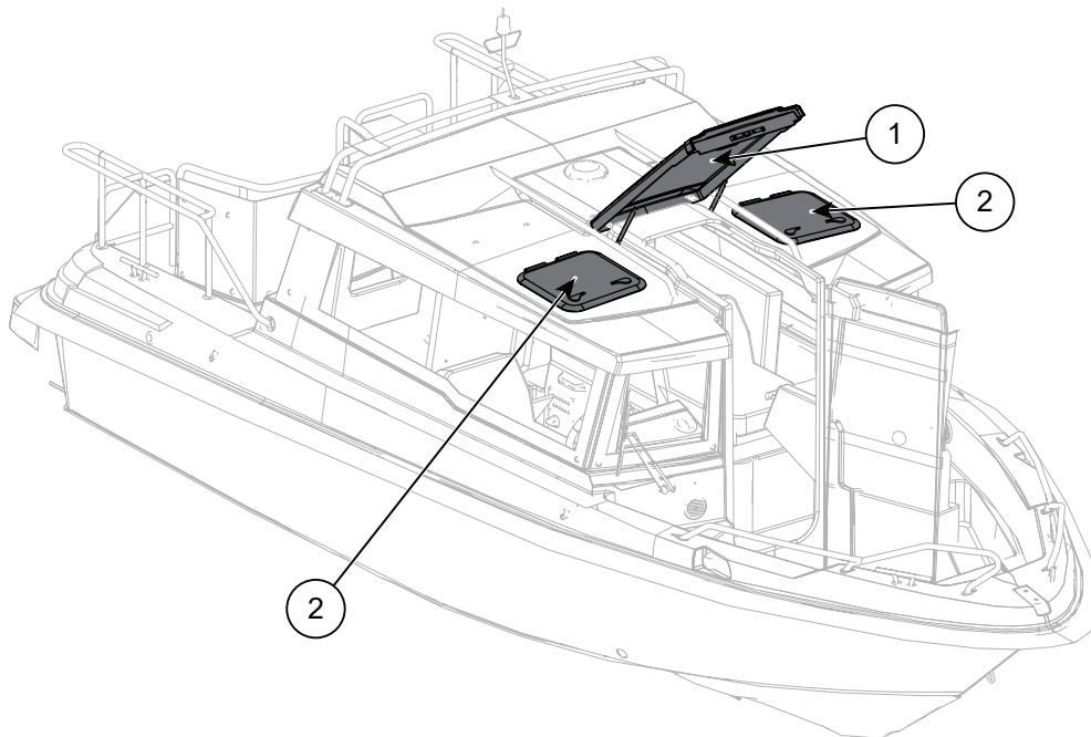
Figur 4.3 Cross 60 Cabin plasseringer av takluker
