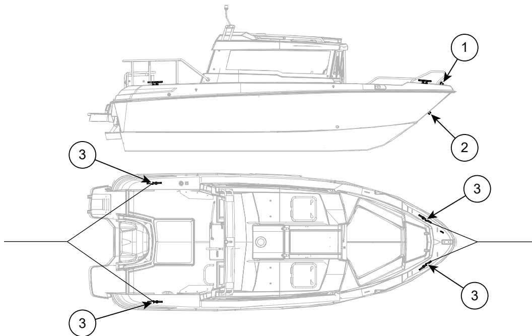
Figur 5.7 Cross 60 Cabin fortøynings- og slepepunkter
